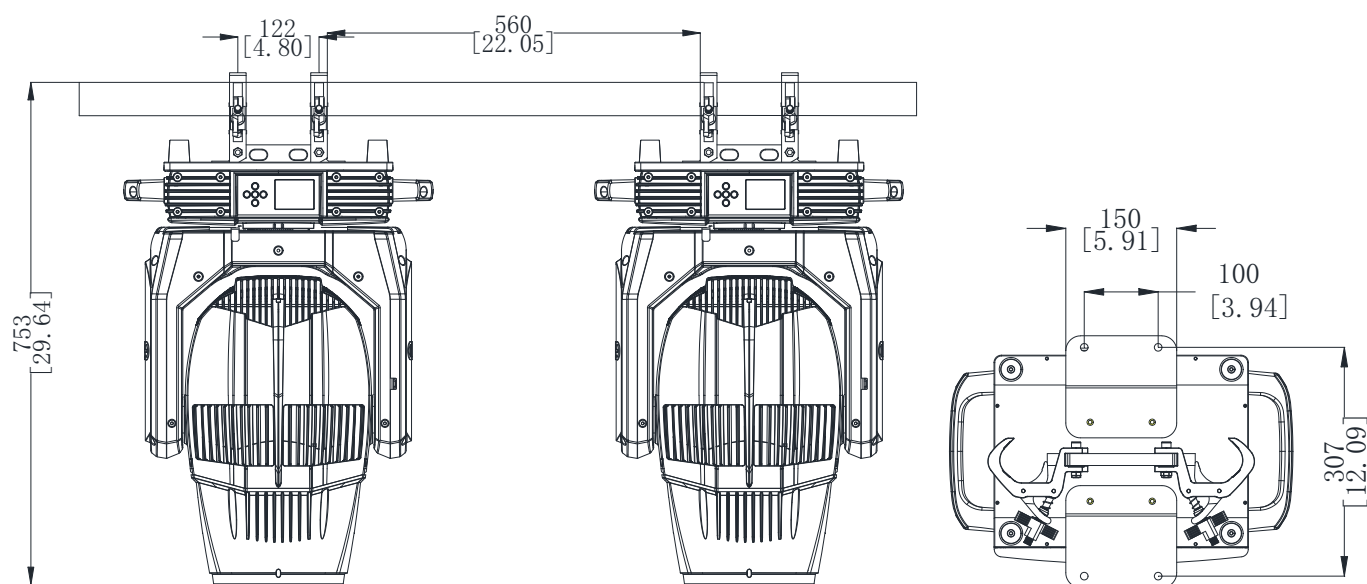
地面安装示意图
