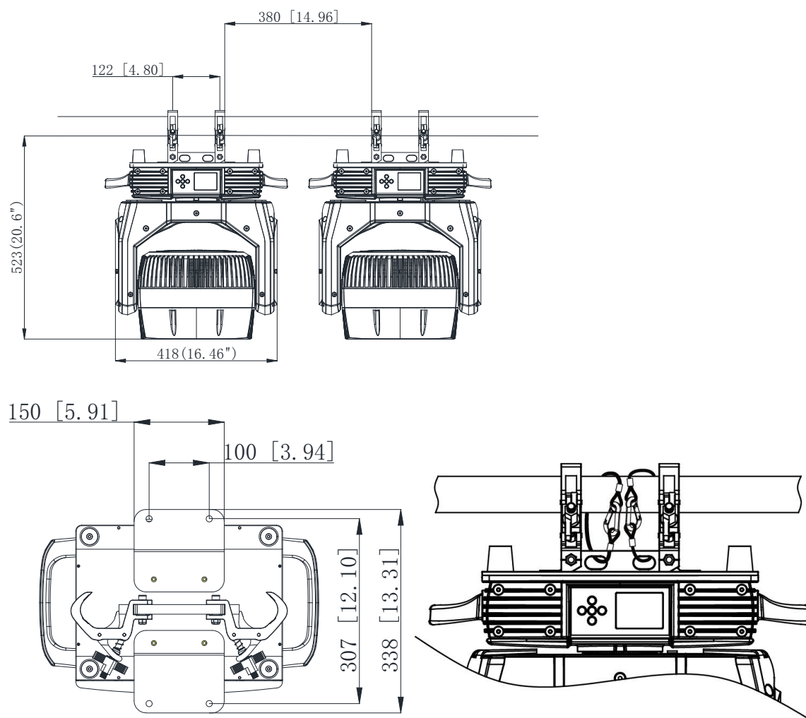
地面安装示意图
